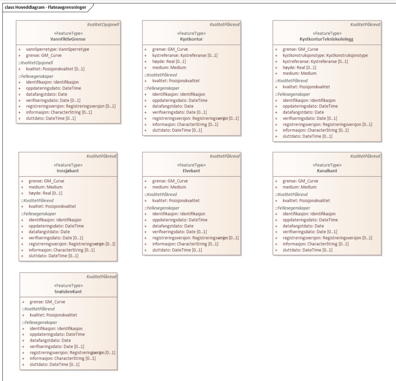
Figur 5. Hoveddiagram - Flateavgrensninger
