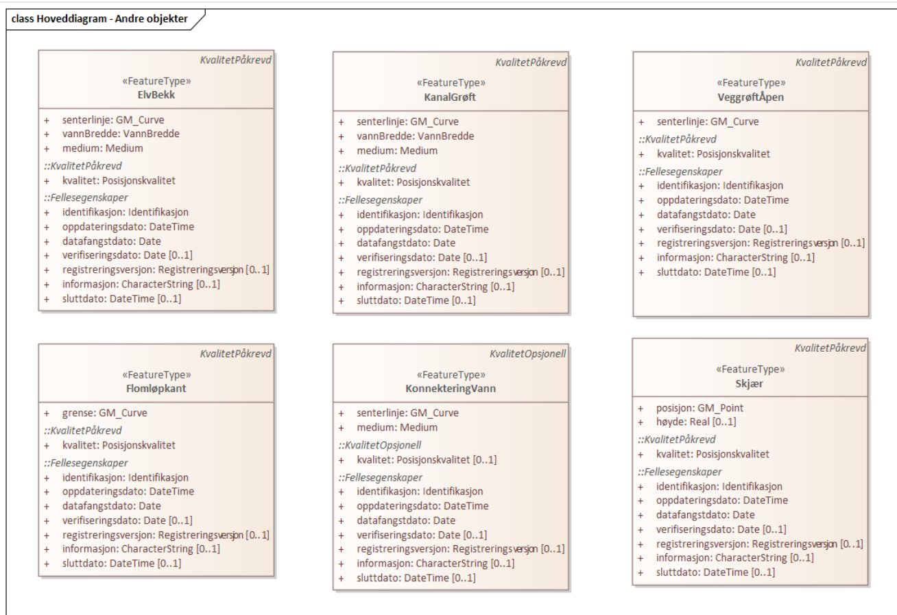
Figur 6. Hoveddiagram - Andre objekter
